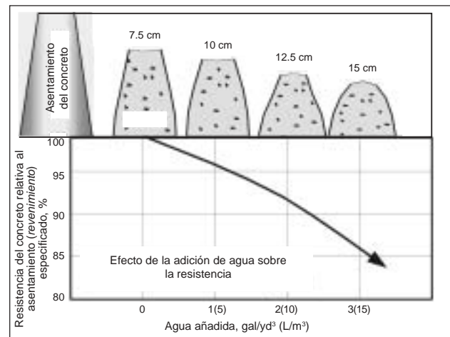
Figura 1. Ejemplo del efecto de la adición de agua sobre el asentamiento y la resistencia del concreto.
